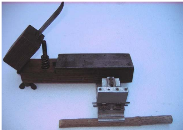
Obr.č.10 Košíkársky hoblík od J Adamčika „otvorený“. Konzola s nožom je odpružená a šírka štrbiny sa reguluje krídlovou maticou,
