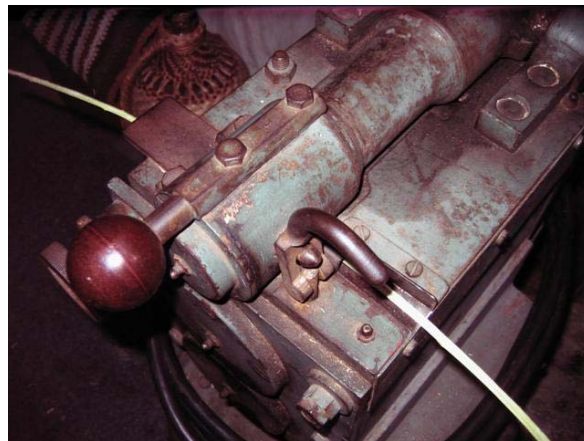
Obr.č. 11 Mechanický hoblík na prúty. Sprava sa vkladajú štiepky, motor si ich ťahá, v ľavo vychádza lubok
